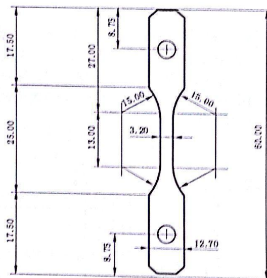
图 D.2 试样的尺寸图
