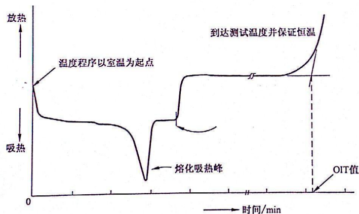
图 F.1 试验温度曲线图
