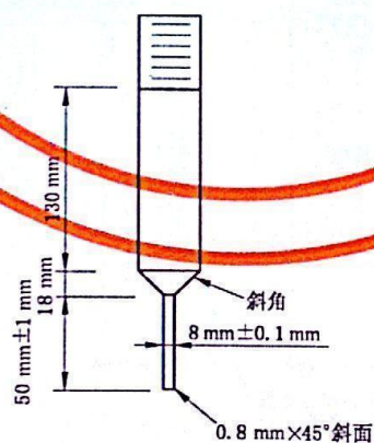
图 C.3 试验穿刺针示意图(未按比例)
